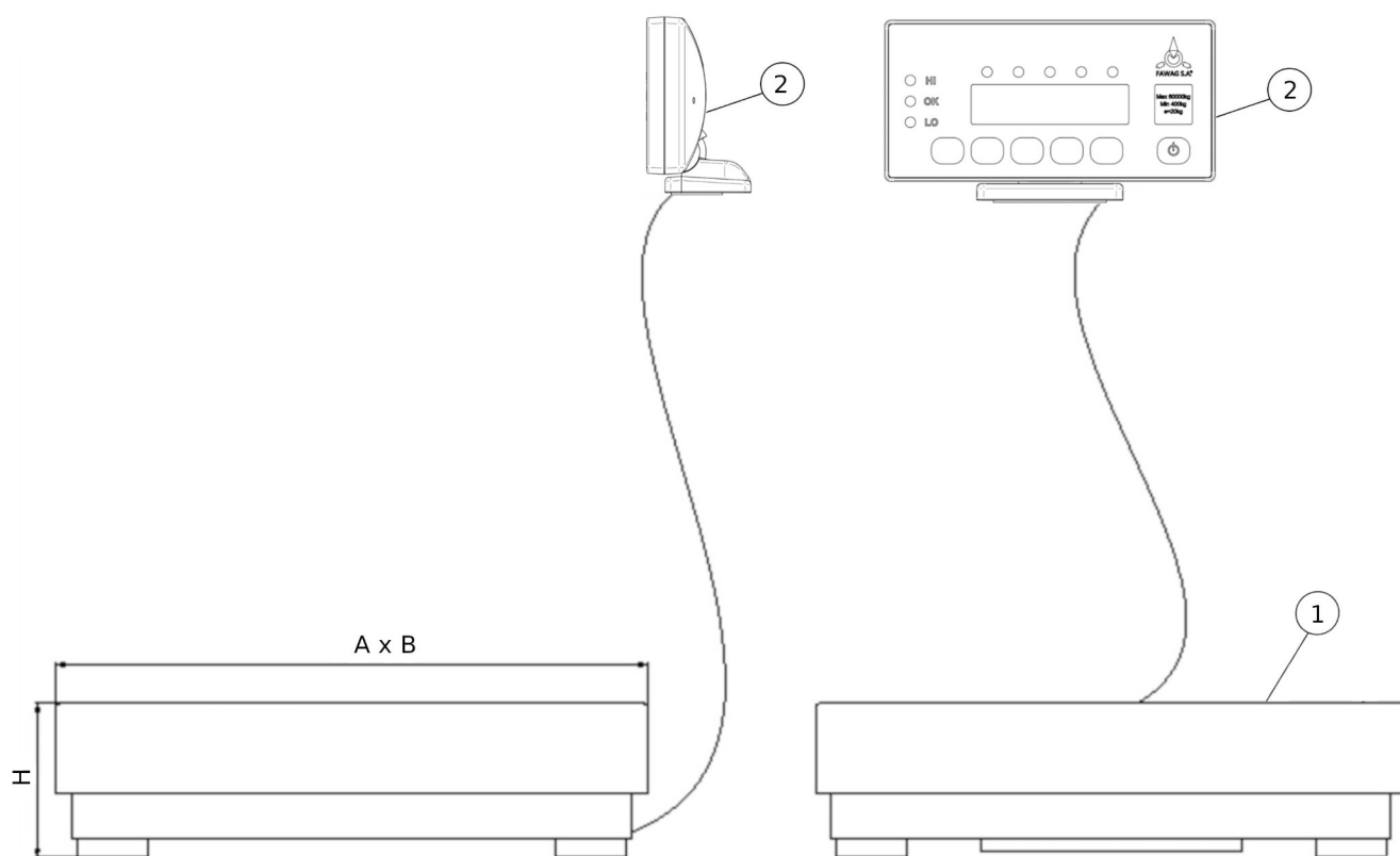
Rys. 1. Wagi WIN 1/1÷WIN 1000/1 wer. A 1-pomost, 2-miernik, 3-pokrętko, 4-kolumna, 5-uchwyt kabla przetwornika
