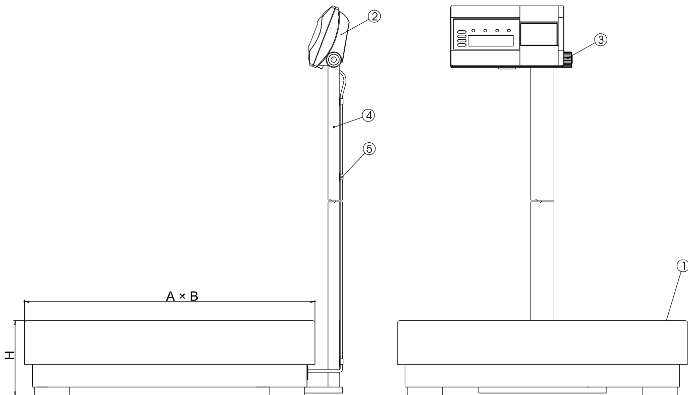
Rys. 1. Wagi WIN 1/1÷WIN 1000/1 wer. A 1-pomost, 2-miernik, 3-pokrętko, 4-kolumna, 5-uchwyt kabla przetwornika
